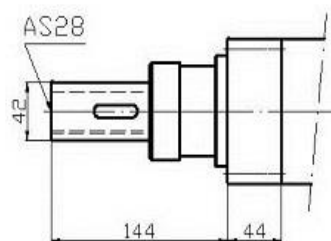
FD67SS-85-AS28
